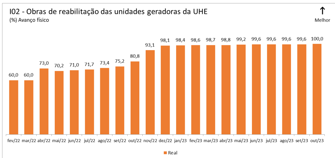
Gráfico 2 - Obras de reabilitação das unidades geradoras da UHE. Gráfico Acumulado*. *Evolução de responsabilidade do Consórcio Candonga (vide nota 2).
