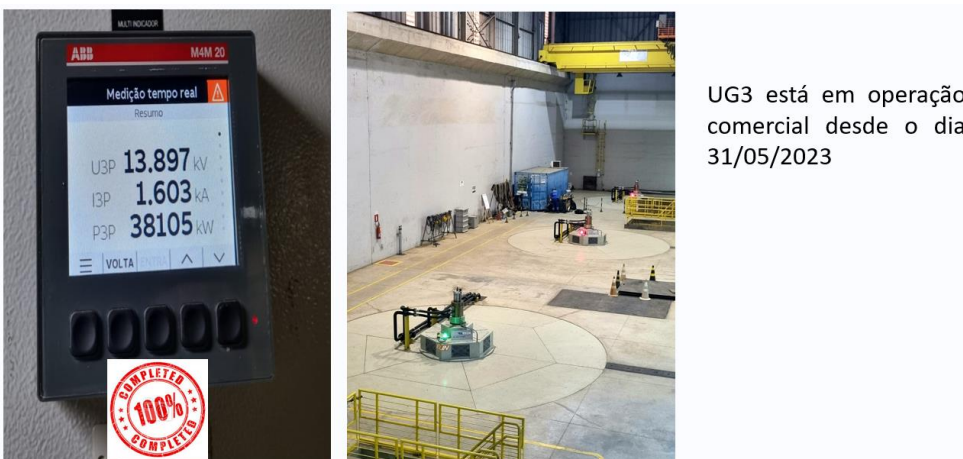
Figura 8 - Dados reabilitação UG3
