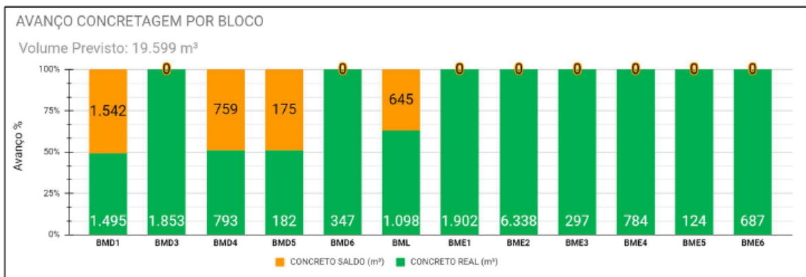
Figura 16 – Avanço concretagem por bloco (Vol. Real. Acum.: 15.898 m 3 )
