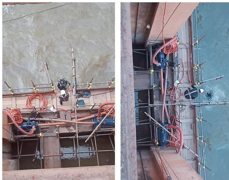
Figura 16 - Mergulho para limpeza de sedimentos e detritos dos túneis de saída d'água Comporta UG1 e ranhuras da UG3
