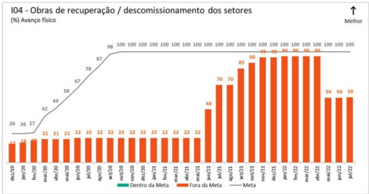
Gráfico 4 - Avanço físico das obras de recuperação / descomissionamento
