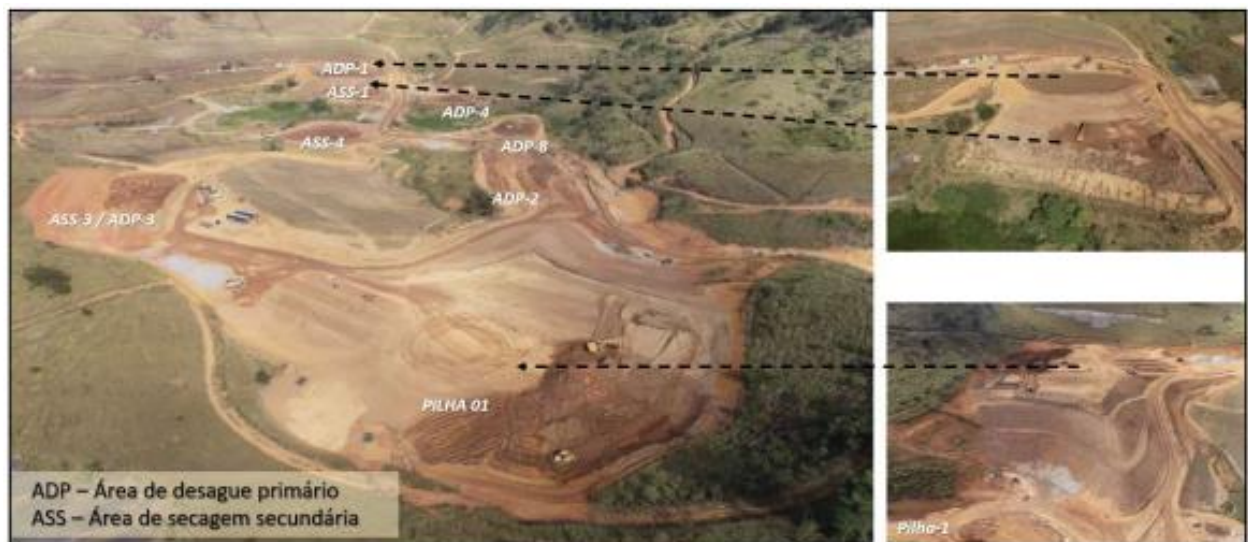
Figura 6 - Foto aérea das área de desaguamento primário e secundário do Setor 11
