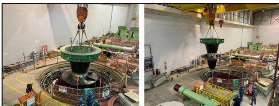
Figura 19 - Recuperação das Unidades de Geração - Rotor Kaplan
