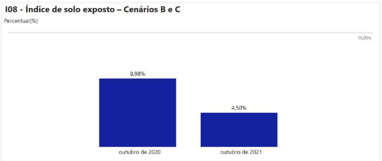
Gráfico 1: I08 - Índice de solo exposto – Cenários B e C - Frequência Bianual
