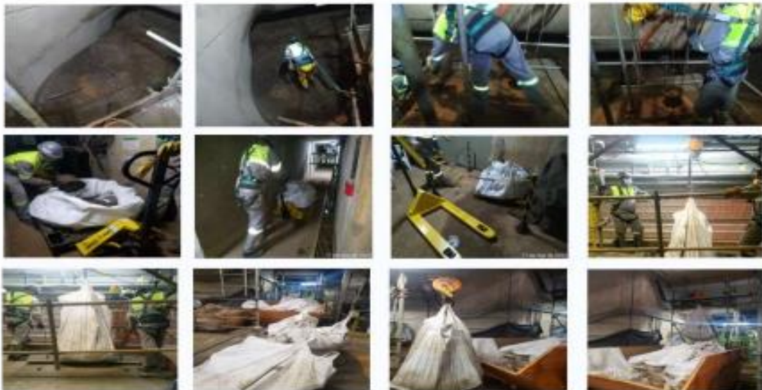
Figura 10 - Teste do hidrojato dentro da UG1, Área de Armazenamento de sedimentos (big bag) e Montagem de Plataforma de Andaime
