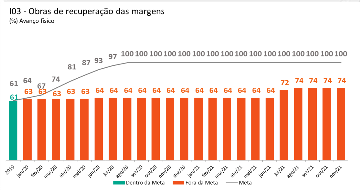
Figura 36 - Gráfico 3. Avanço físico das obras de recuperação das margens. Gráfico Acumulado.
