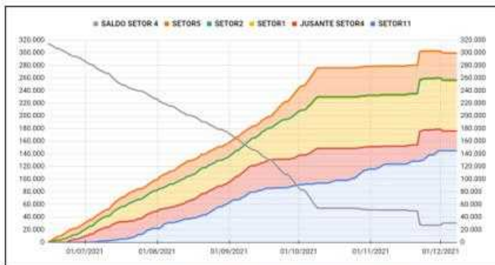
Figura 3 - Gráfico de Disposição de Sedimentos
