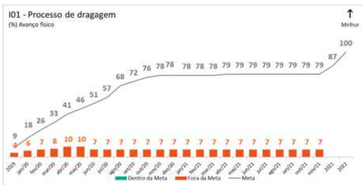
Figura 34 - Gráfico 1. Avanço físico do processo de dragagem. Gráfico Acumulado.
