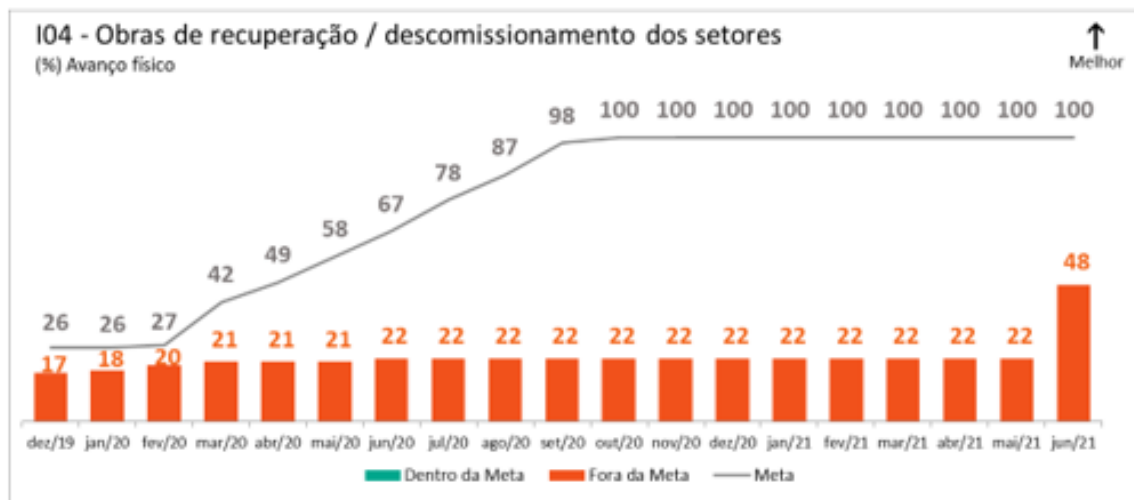
Gráfico 4. Avanço físico das obras de reabilitação / descomissionamento dos setores. Gráfico Acumulado.
