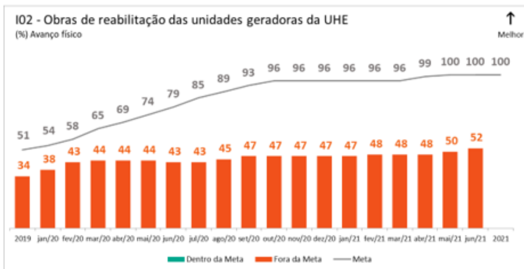
Gráfico 3. Avanço físico das obras de reabilitação das unidades geradoras da UHE. (Gráfico Acumulado).
