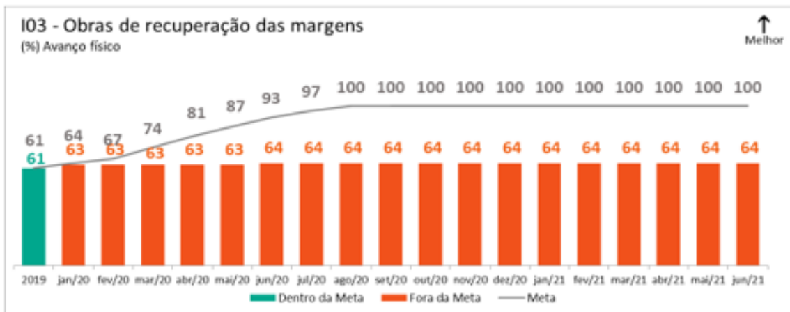
Gráfico 3. Avanço físico das obras de recuperação das margens. Gráfico Acumulado.
